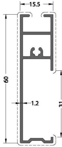
horizontalframeprofile dişiray
