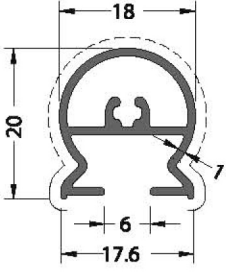
frontframeprofile önpanoprofil
