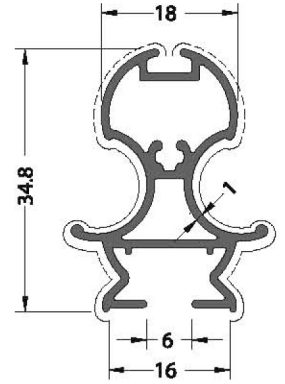
flatconnectionsashprofile düzmıknatıslıprofil
