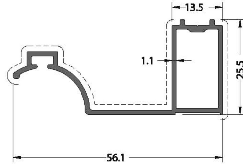
sash closing adapter for 2 sash detail çiftçalışırılık karşılık
