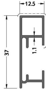
horizontalframeprofile ray
