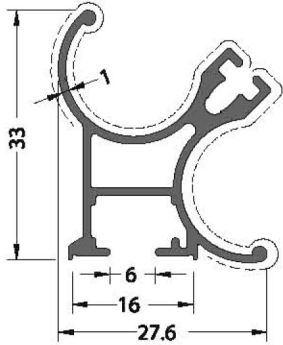
angularconnectionsashprofile köşemıknatıslıprofil
