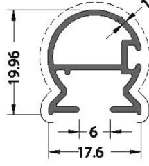
backsashprofile arkakanatprofil
