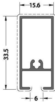
horizontalsashprofile yataykanatprofil
